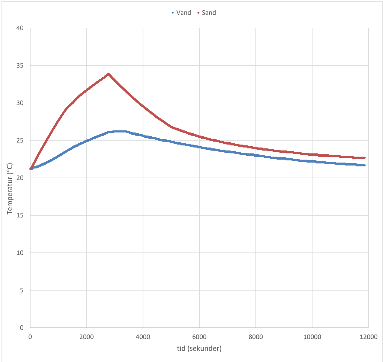
Figur 1: Temperaturens ændring over tid i to materialer opvarmet med en varmelampe.
